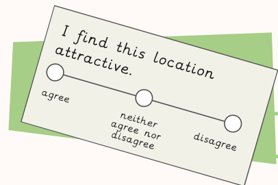
Likert scales
